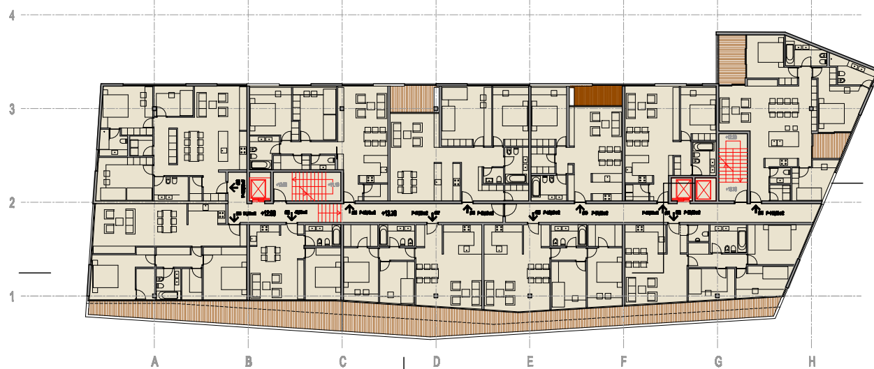
TLOCRT 4. KATA 1 : 200
