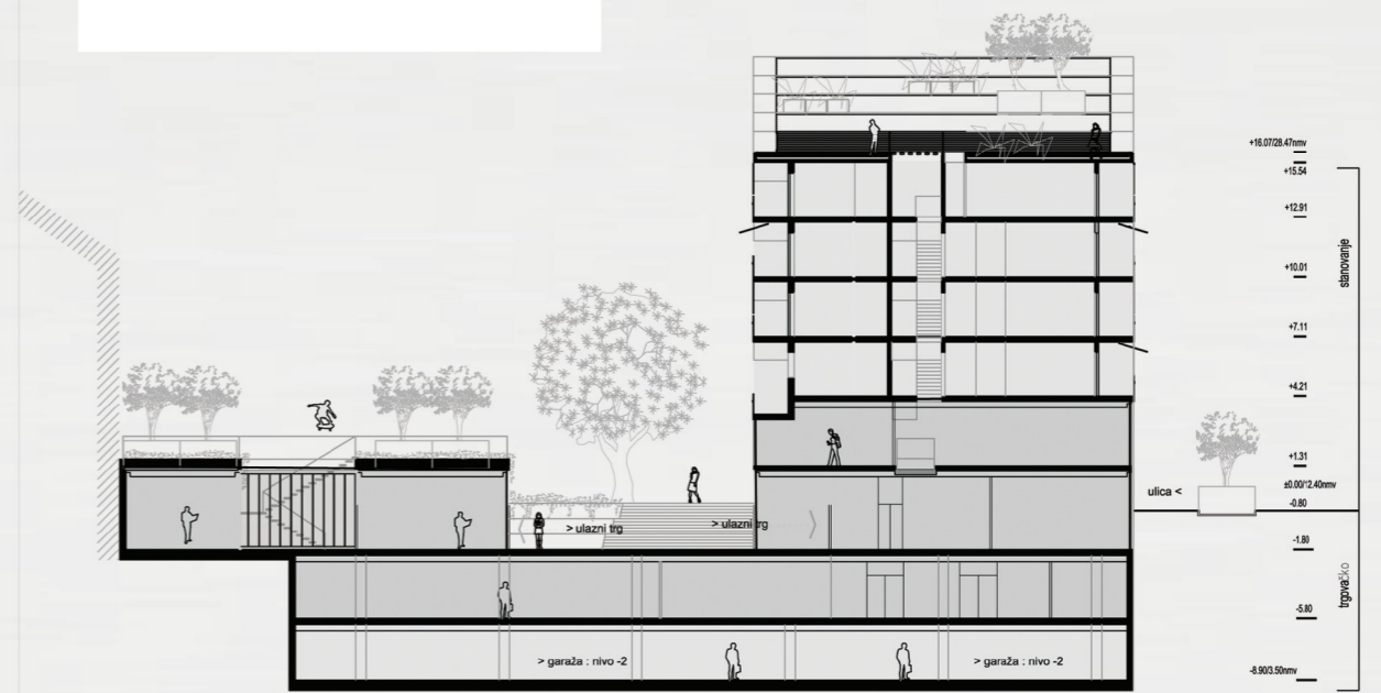
:: poprečni presjek B-B
